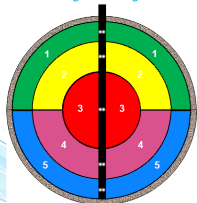
Die Anordnung der Sensorpaare repräsentiert flächengleiche Segmente
